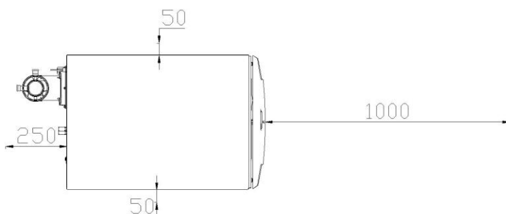
Figura 11: Spazi di installazione (mm)
