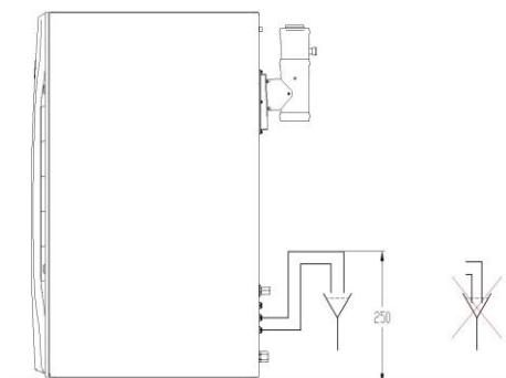
Figura 17: altezza massima dello scarico del troppo pieno
