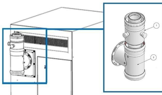
Figura 25: Connettore scarico fumi BLUEGEN BG-08
