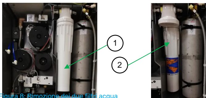
Figura 8: Rimozione dei due filtri acqua
