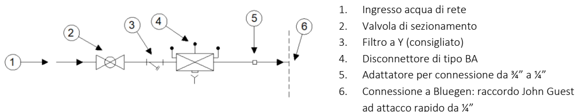
Figura 16: Configurazione consigliata della connessione di alimentazione dell'acqua
