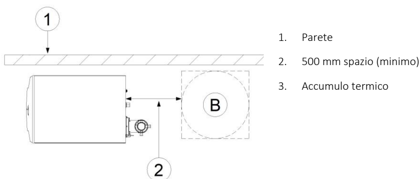
Figura 12: Spazio tra BLUEGEN BG-08 e accumulo termico
