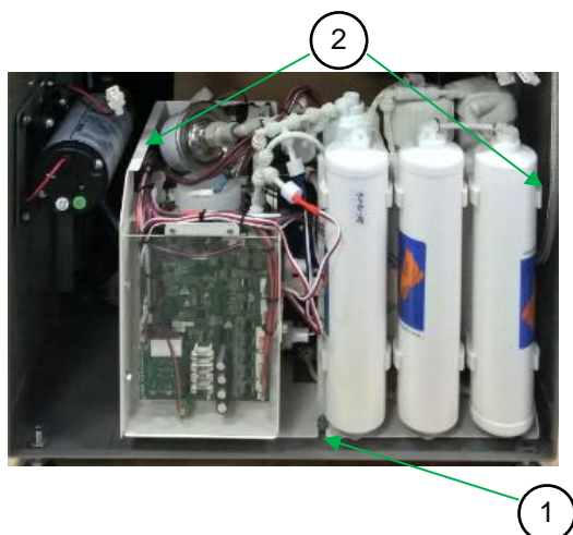
Figura 7: Sistema di trattamento dell'acqua (WTS)
