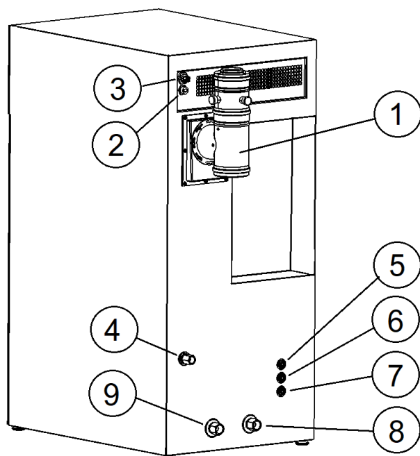
Figura 2: Connessioni esterne al sistema
