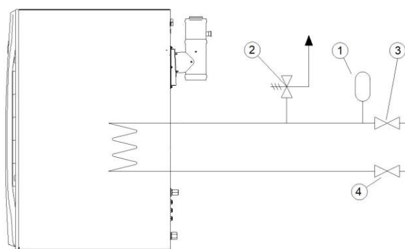
Figura 24: Configurazione circuito per isolamento del recupero termico
