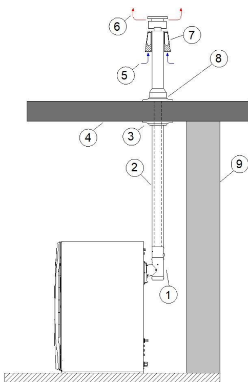
Figura 27: installazione condotto con terminale verticale (Tipo C33)
