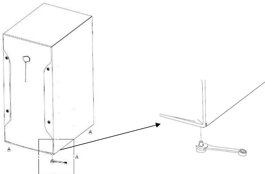
Figura 14: Piedini di montaggio regolabili
