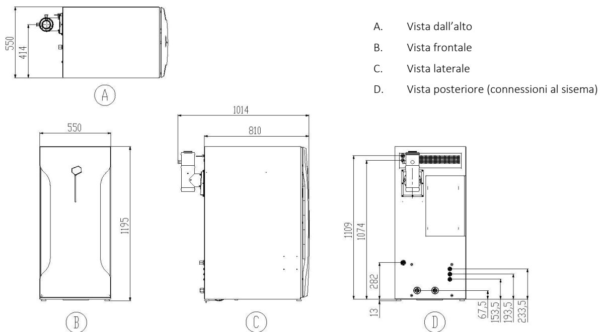
Figura 3: Dimensioni del BLUEGEN BG-08 (mm)
