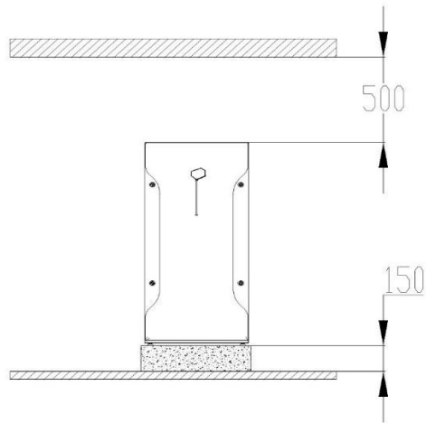
Figura 13: Spazi minimi tra BLUEGEN BG-08 e strutture permanenti
