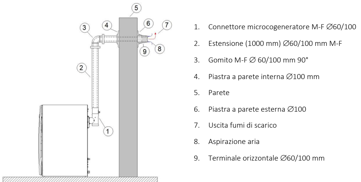
Figura 26: Installazione uscita a parete (Tipologia C13)
