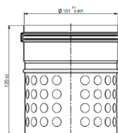
Figura 30: Presa d'aria
