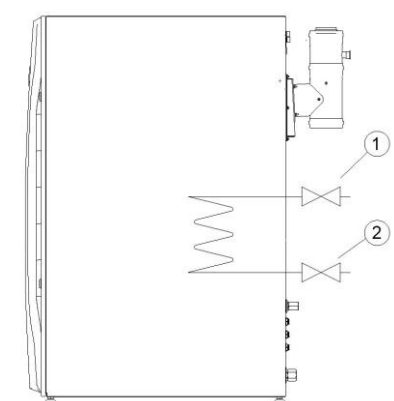
Figura 23: Configurazione circuito per isolamento del recupero termico
