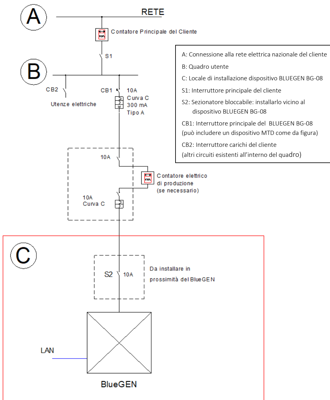
Figura 18: Installazione elettrica
