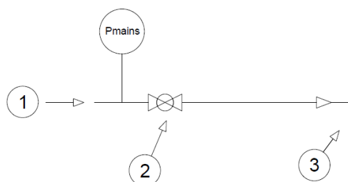
Figura 15: Condotto gas consigliato con valvola regolatrice di pressione.
